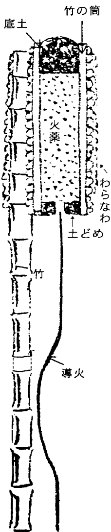
図 龍勢の構造
